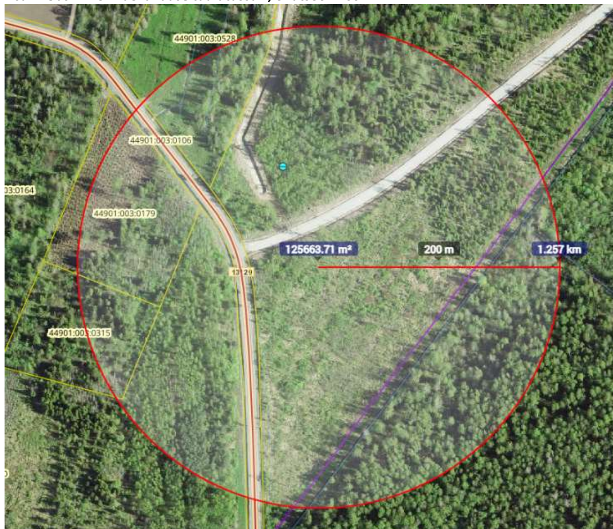
Lisa 1. Uus-Kiviõli kaevanduse tuulutusšurf, ohutsoon 200 m
